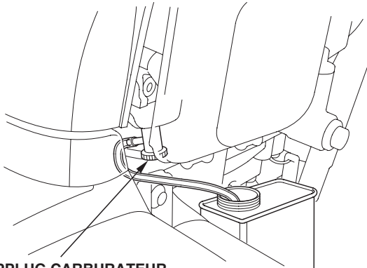
AFTAPPLUG CARBURATEUR
