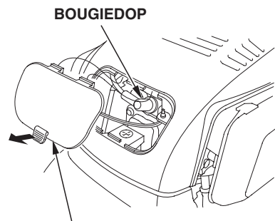
CONTROLELUIKJE
