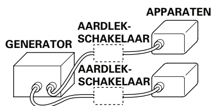
Aansluiting op twee aardlekschakelaars
